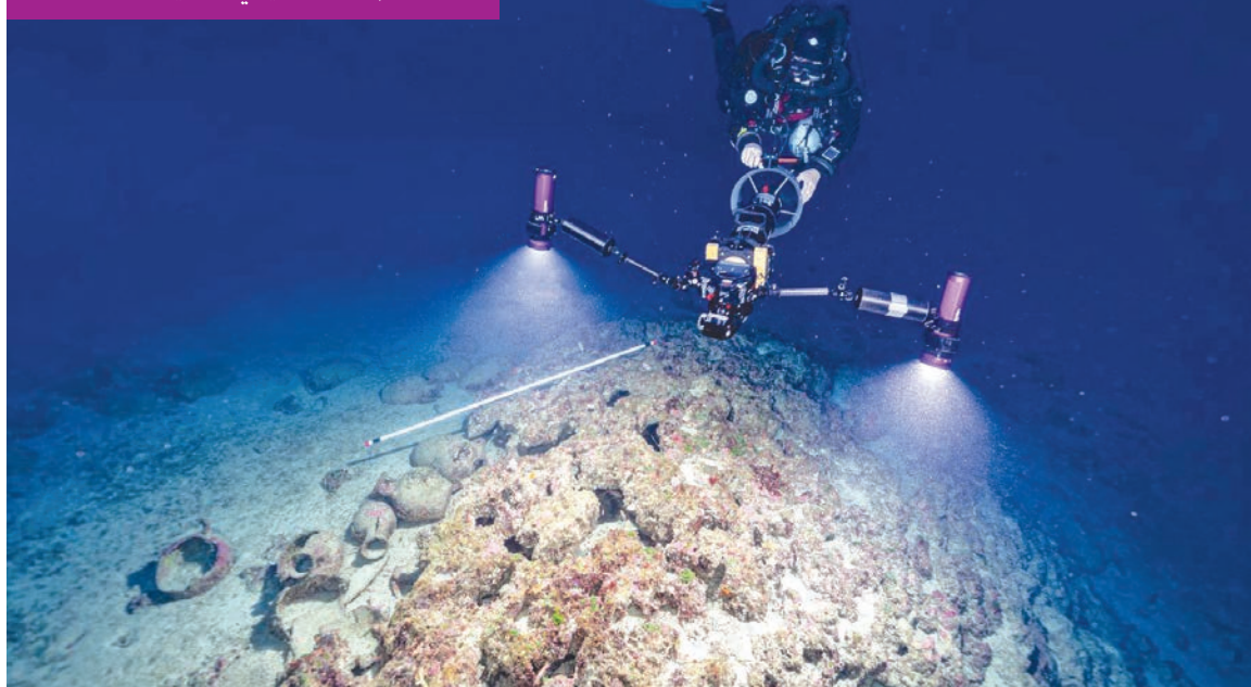
التصوير المساحي ثلاثي الأبعاد تحت الماء (الصورة بإذن من د. تيمى غامبين)
